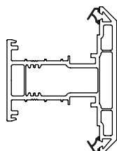
Transom 'T' ERW31
